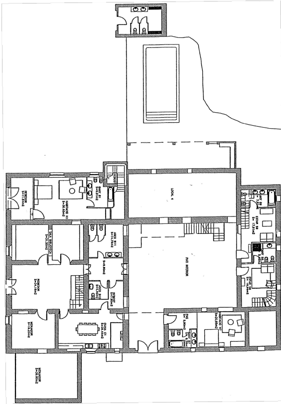
PLANTA BAJA
